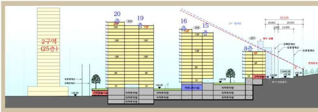
A-A' 단 면 도 (특별건축구역 지정안)
