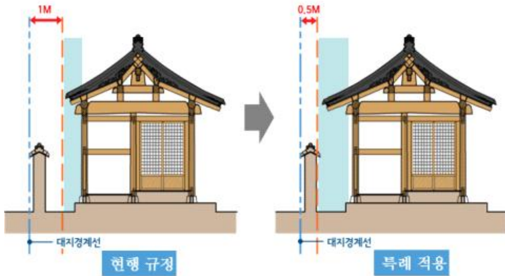
전통적 조경기법 구현을 위한 대지의 조정 완화
